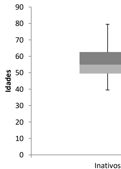
BOXPLOT INATIVOS
